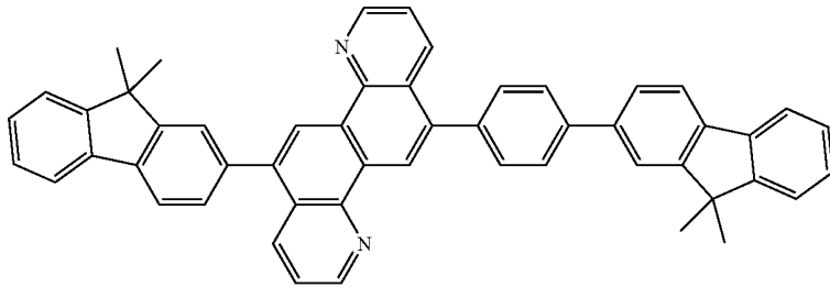
[Chem. 6]
